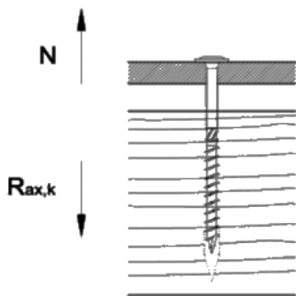
Odpor na ťah ocel' - drevo R_{ax,k} [kN]
