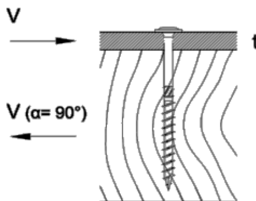
Strih ocel' - drevo R_k [kN]
